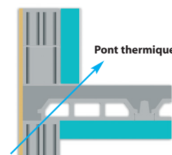
Plancher conventionnel
